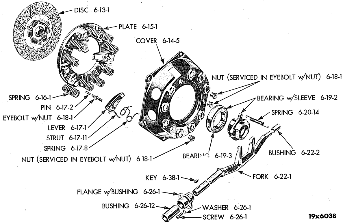
CLUTCH
